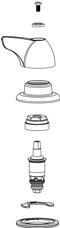
Short Stem Cartridge / Cartucho de barra corta / Cartouche avec tige courte
